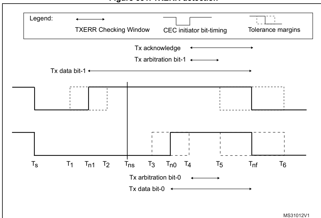
Figure 531. TXERR detection
